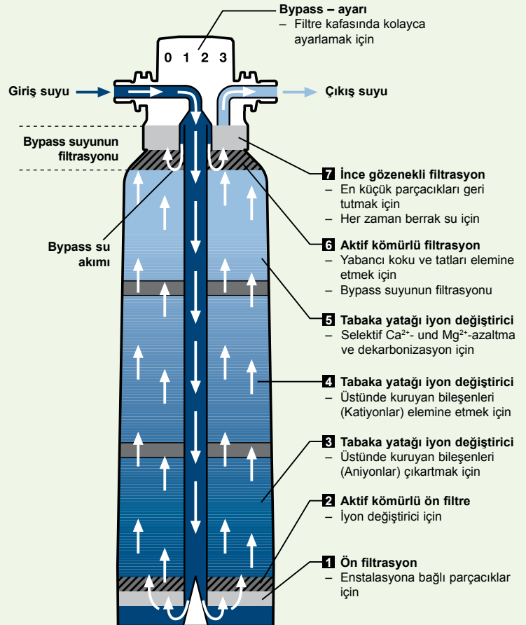
7-defa filtrasyonlu bir BWT bestclear EXTRA filtre kartuşunun yapısı
