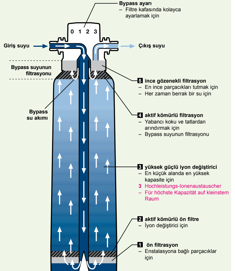
5-defa filtrasyonlu bir BWT bestclear filtre kartuşunun yapısı
