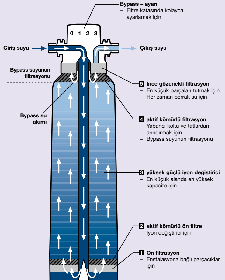
5-defa filtrasyonlu bir BWT bestprotect filtre kartuşunun yapısı
